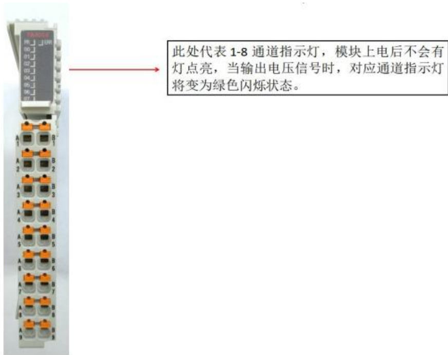
图3-8 FA40C8/FA42C8 指示灯说明
