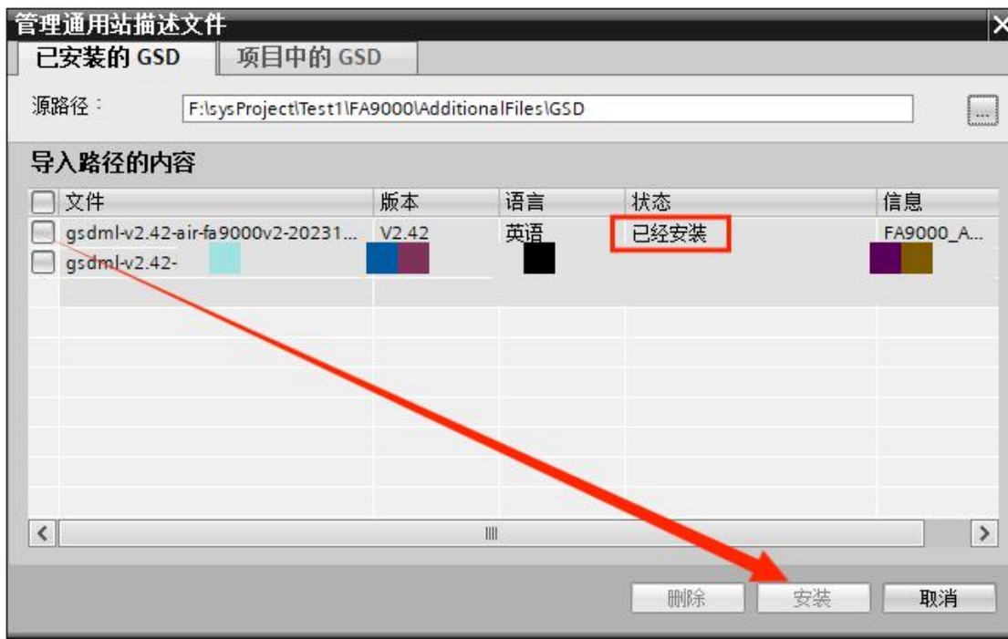
图4-10 添加GSD
