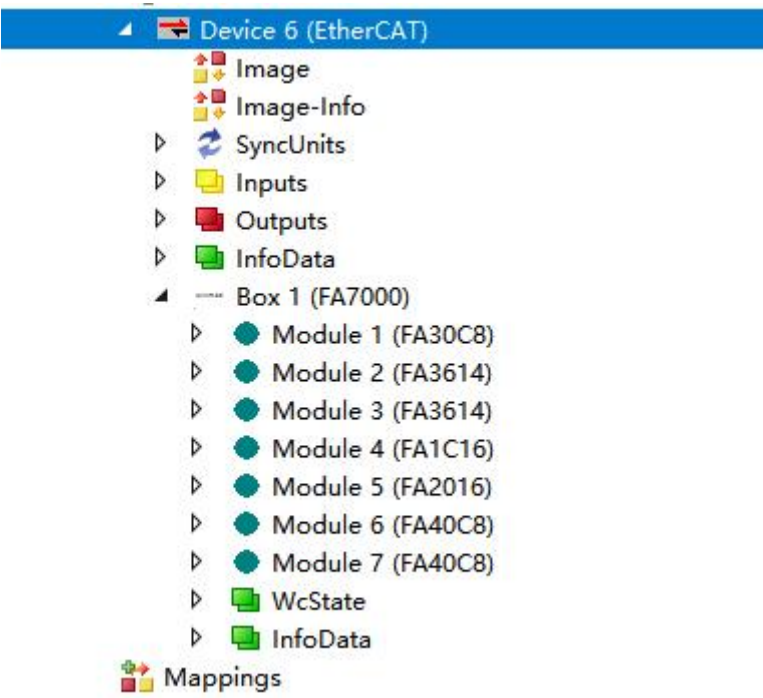
图4-6 硬件组态
