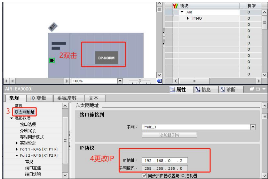
图4-14 分配IP地址
