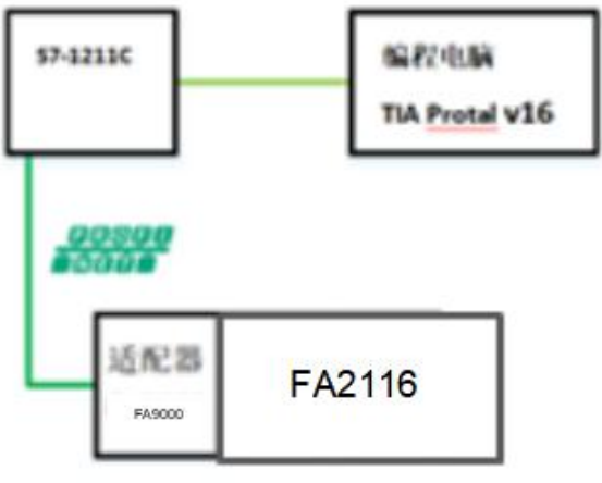
图4-8 通信连接图
