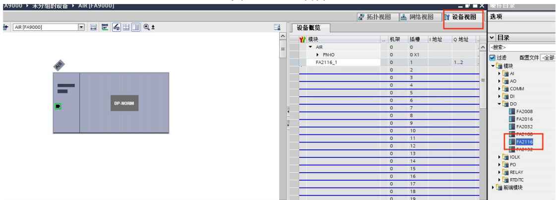
图4-12 组态I/O模块
