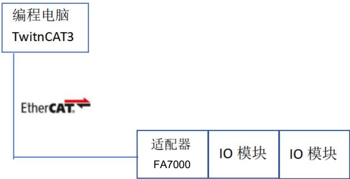
图4-1通信连接图
