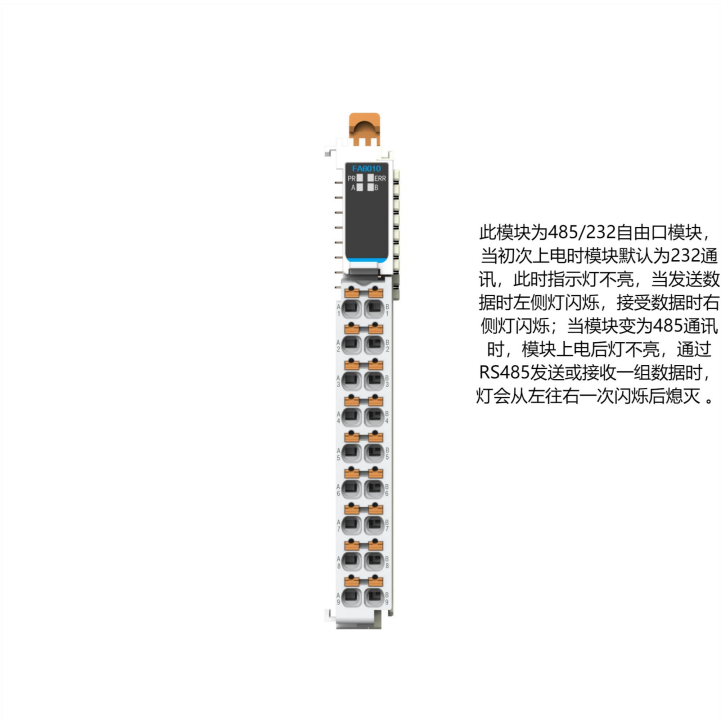
图 3-2 FA6010 电源指示
