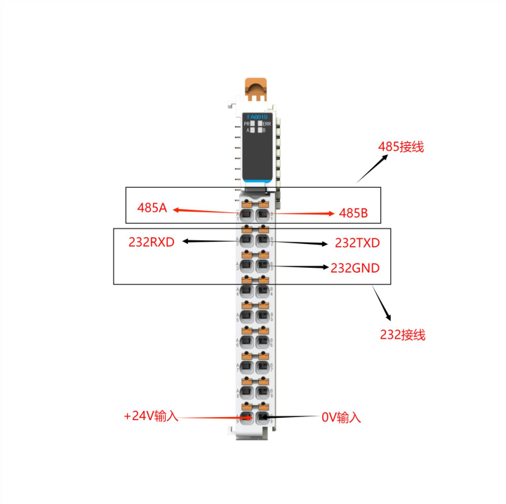
图3-1 FA6010 接线图
