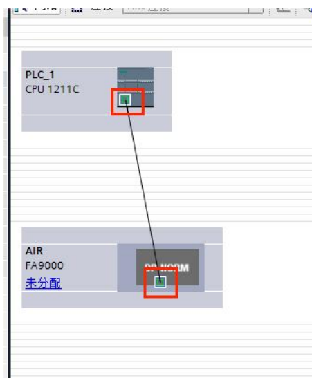
连接 PLC 与 FA9000 方法二
