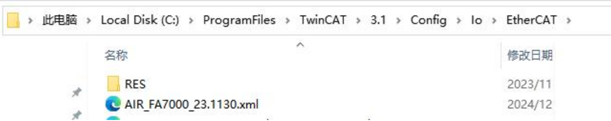
图5-2 安装XML描述文件
