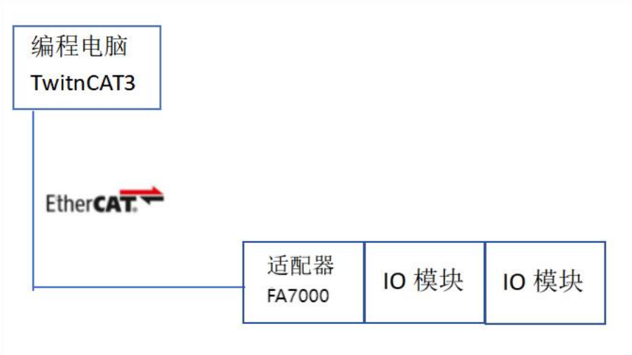
图5-1 通信连接图
