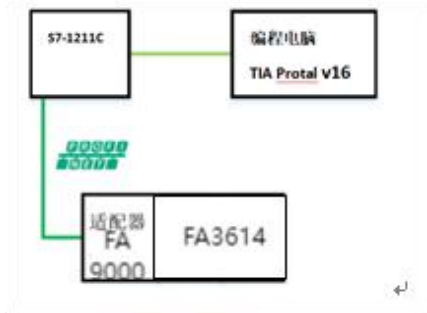
图4-9 通信连接图
