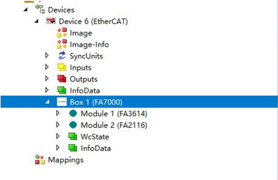
图4-6硬件组态
