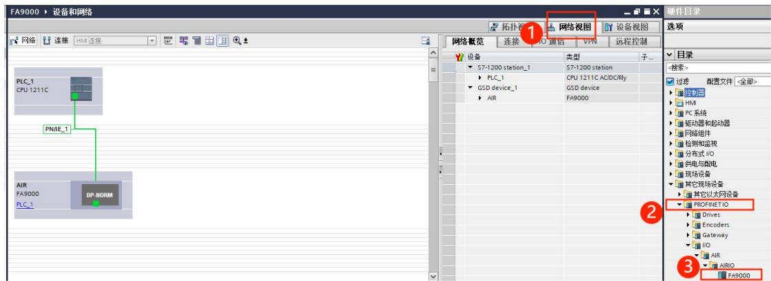
图4-11 组态设备
