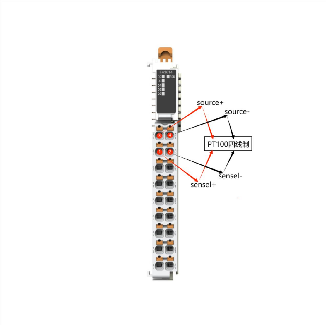
图3-3 四线制接线图
